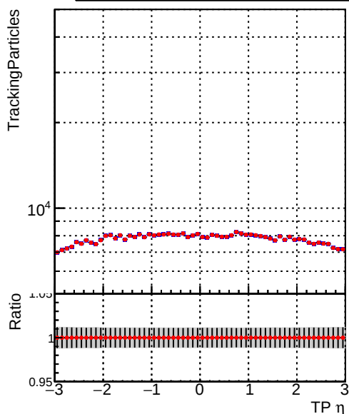
DQM_TT_ORIGINAL DQM_TT_MODIFIED_propToPlane_PRVersionFINAL5
