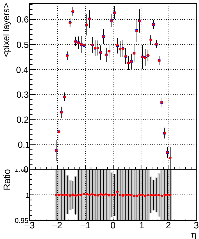
Legend: ■ DQM_TT_ORIGINAL ● DQM_TT_MODIFIED_propToPlane_PRVersionFINAL5
