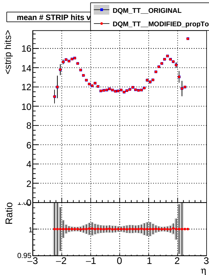
Legend: ■ DQM_TT_ORIGINAL ● DQM_TT_MODIFIED_propToPlane_PRVersionFINAL5
