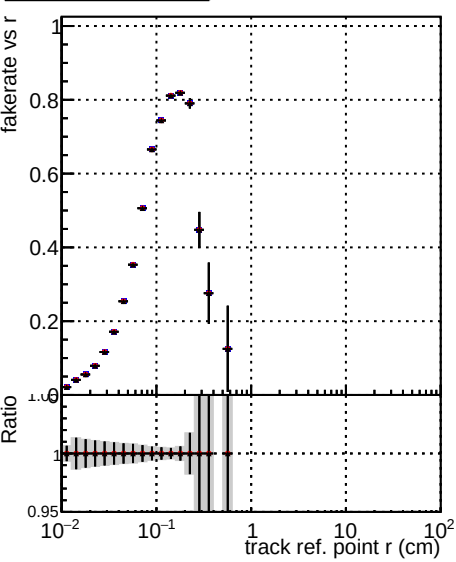
—•— DQM TT ORIGINAL —•— DQM TT MODIFIED propToPlane_PRRVersionFINAL2 —•— DQM TT MODIFIED propToPlane_PRRVersionFINAL4
