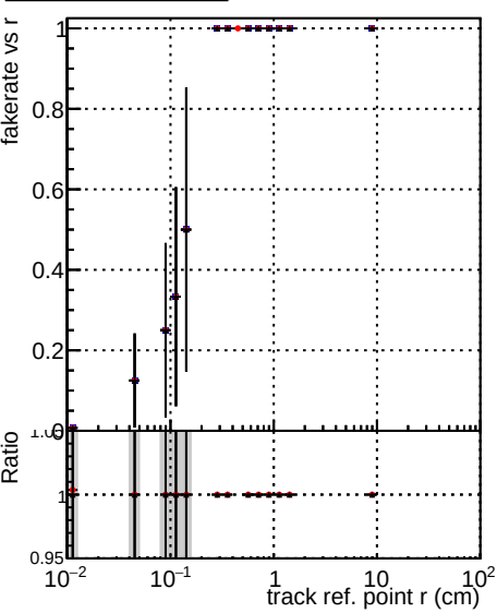
Fake rate vs verpos DQM TT ORIGINAL DQM TT MODIFIED DQM TT MODIFIED propToPlane_PRVersionFINAL2 DQM TT MODIFIED propToPlane_PRVersionFINAL4
