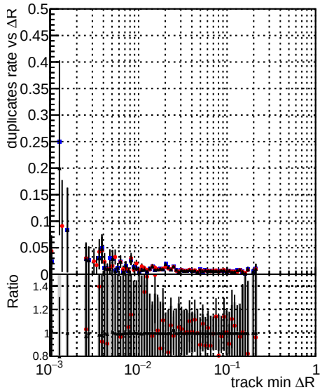
—●— DQM TT ORIGINAL —●— DQM TT MODIFIED —●— DQM TT MODIFIED propToPlane_PRRVersionFINAL2
