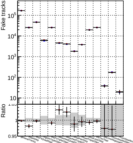
Number —■— DQM_TT_ORIGINAL —●— DQM_TT_MODIFIED_propToPlane_PRVersionFINAL2 —▲— DQM_TT_MODIFIED_propToPlane_PRVersionFINAL3
