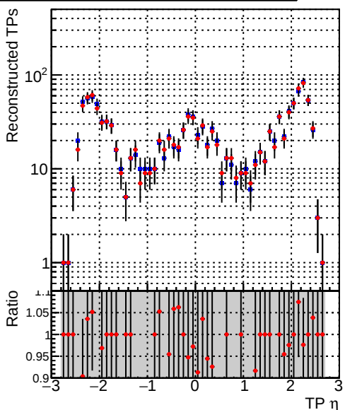
—●— DQM_TT_ORIGINAL —●— DQM_TT_MODIFIED_propToPlane_PRVersionFINAL2
