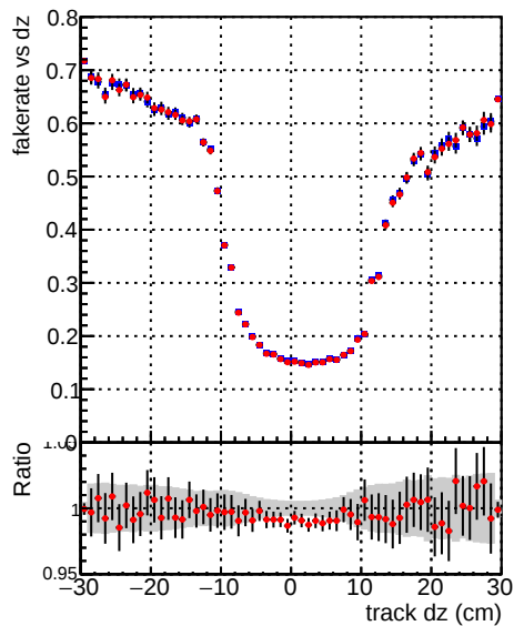
Fake rate vs dz —●— DQM TT ORIGINAL —●— DQM TT MODIFIED_propToPlane_PRVersionFINAL2
