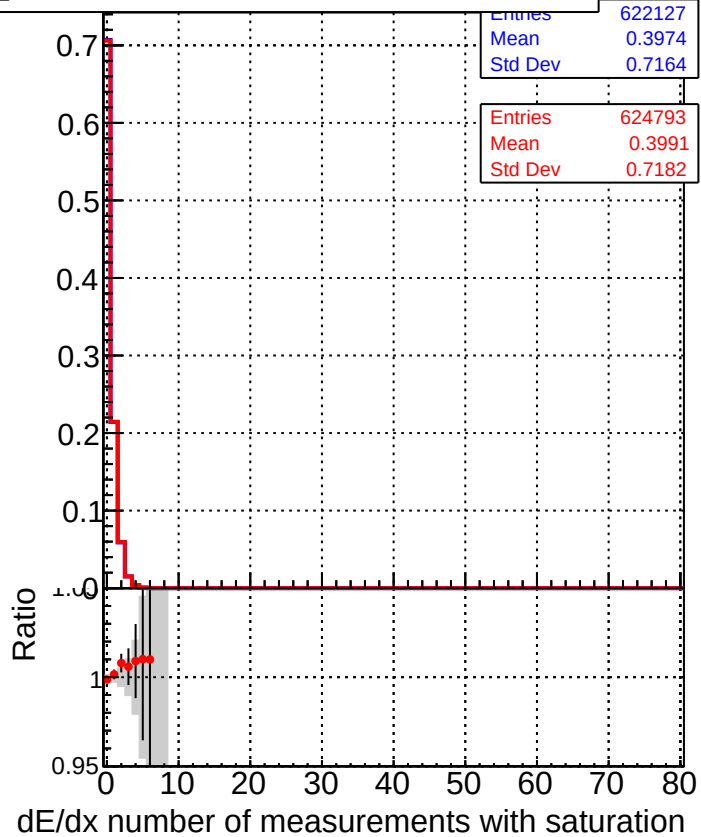
■ DQM_TT_ORIGINAL ● DQM_TT_MODIFIED_propToPlane_PRVersionFINAL2
