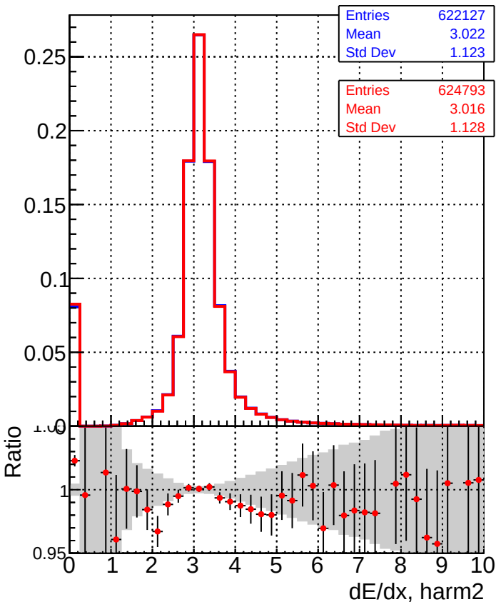
■ DQM_TT_ORIGINAL ● DQM_TT_MODIFIED_propToPlane_PRVersionFINAL2
