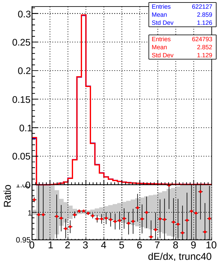
■ DQM_TT_ORIGINAL ● DQM_TT_MODIFIED_propToPlane_PRVersionFINAL2
