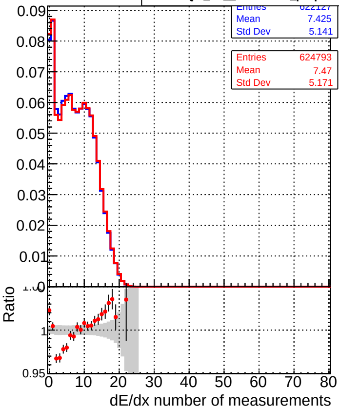
■ DQM_TT_ORIGINAL ● DQM_TT_MODIFIED_propToPlane_PRVersionFINAL2
