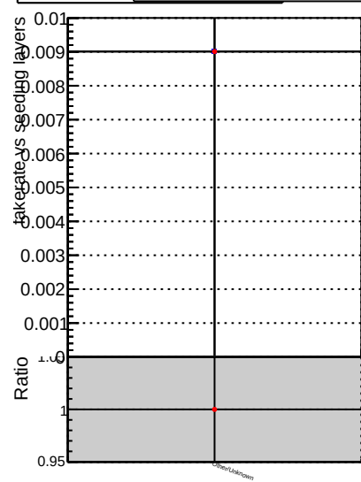
Fake rate vs. DQM TT ORIGINAL DQM TT MODIFIED propToPlane_PRVersionFINAL2
