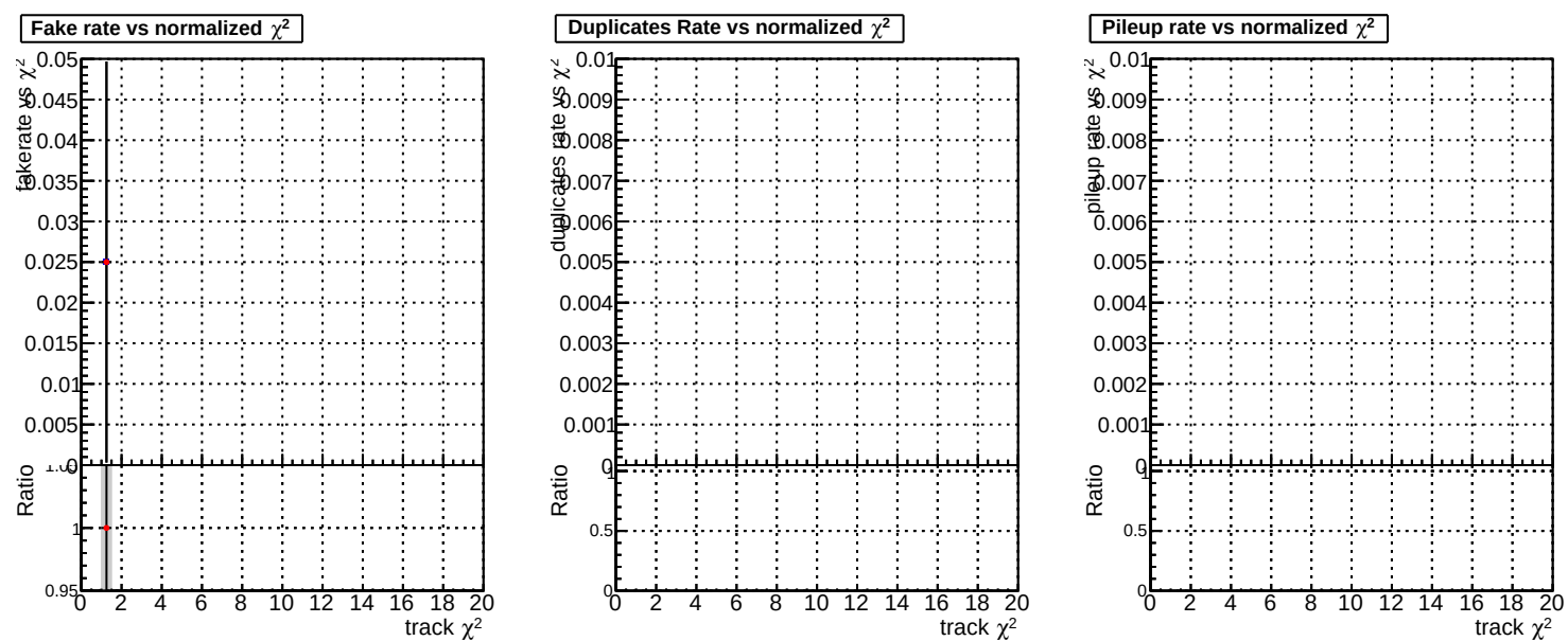
Fake rate vs. DQM TT ORIGINAL DQM TT MODIFIED propToPlane_PRVersionFINAL2
