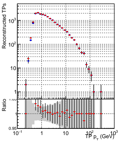
■ DQM_TT_ORIGINAL ■ DQM_TT_MODIFIED_propToPlane_PRVersionFINAL
