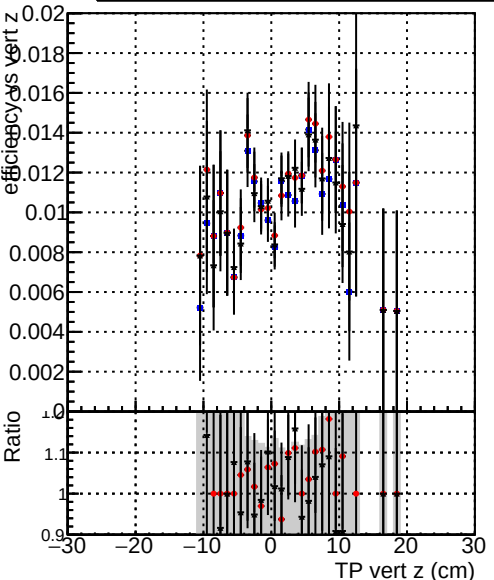
Efficiency vs TP vert z (cm) Legend: DQM_TT_ORIGINAL DQM_TT_MODIFIED_layerProc v2 DQM_TT_MODIFIED_layerProc v2_OctoberVersion
