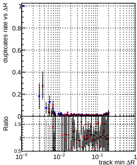
—●— DQM TT ORIGINAL —●— DQM TT MODIFIED —●— DQM TT MODIFIED layerProcv2_OctoberVersion
