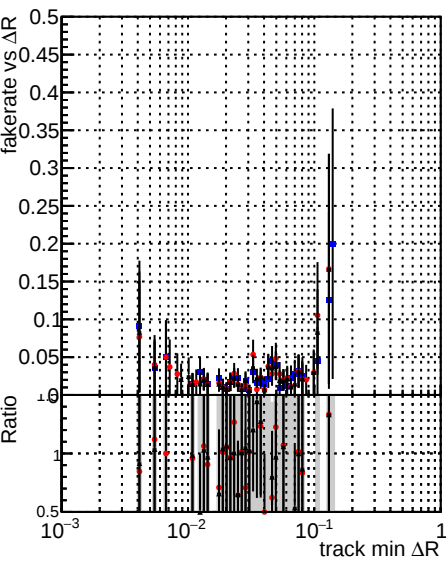
Legend: DQM TT ORIGINAL (black), DQM TT MODIFIED_layerProcv2 (red), DQM TT MODIFIED_layerProcv2_OctoberVersion (blue)
