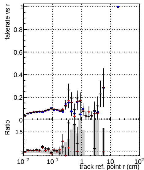
—●— DQM TT ORIGINAL —●— DQM TT MODIFIED_layerProcv2 —●— DQM TT MODIFIED_layerProcv2_OctoberVersion
