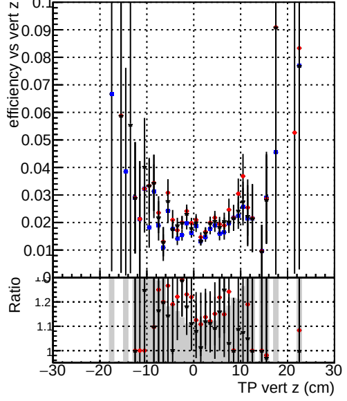
Efficiency vs TP vert z —●— DQM_TT_ORIGINAL —●— DQM_TT_MODIFIED_layerProcV2 —●— DQM_TT_MODIFIED_layerProcV2_OctoberVersion
