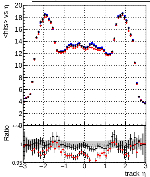
— DQM_TT_ORIGINAL — DQM_TT_MODIFIED_layerProcV2 — DQM_TT_MODIFIED_layerProcV2_OctoberVersion
