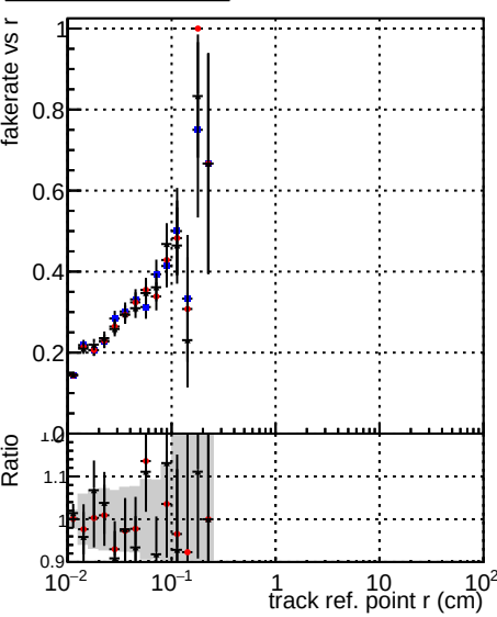
Fake rate vs verpos DQM TT ORIGINAL DQM TT MODIFIED DQM TT MODIFIED layerProcv2 OctoberVersion
