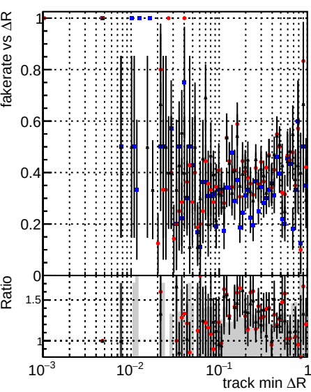
Fake rate vs \Delta R(\text{track, jet}) DQM TT ORIGINAL DQM TT MODIFIED DQM TT MODIFIED layerProcv2_OctoberVersion
