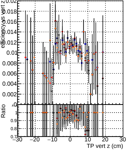
Efficiency vs TP vert z Legend: DQM TT ORIGINAL DQM TT MODIFIED layerProcv2 DQM TT MODIFIED layerProcv2_windows DQM TT MODIFIED layerProcv2_windows_hits
