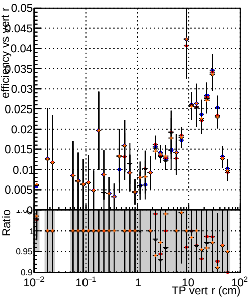
Efficiency vs TP vert r (cm) Legend: DQM TT ORIGINAL DQM TT MODIFIED layerProcv2 DQM TT MODIFIED layerProcv2_windows DQM TT MODIFIED layerProcv2_windows_hits
