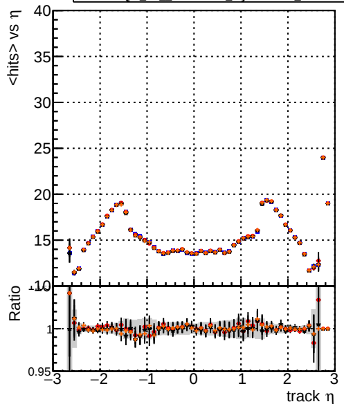
mean hits vs \eta DQM TT ORIGINAL DQM TT MODIFIED layerProcv2 DQM TT MODIFIED layerProcv2_windows DQM TT MODIFIED layerProcv2_windows_hits
