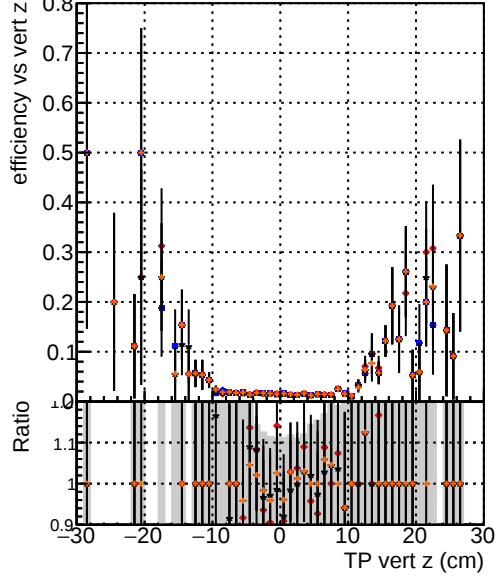
Efficiency vs TP vert z —●— DQM TT ORIGINAL —●— DQM TT MODIFIED layerProcv2 —●— DQM TT MODIFIED layerProcv2_windows —●— DQM TT MODIFIED layerProcv2_windows_hits
