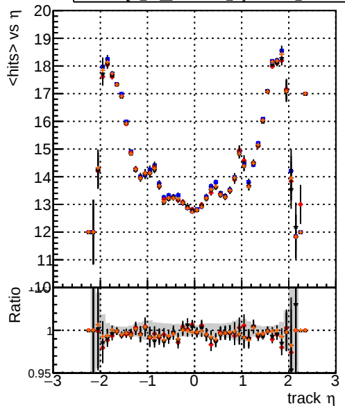
mean hits vs \eta Legend: DQM TT ORIGINAL layerProc2 DQM TT MODIFIED layerProc2 DQM TT MODIFIED layerProc2_windows DQM TT MODIFIED layerProc2_windows_hits
