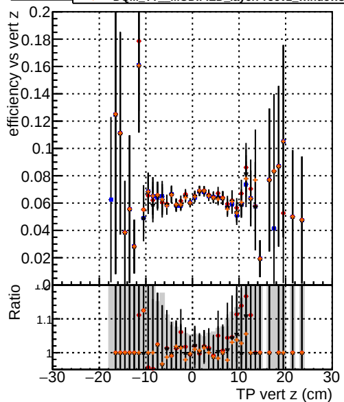
Efficiency vs vert z —●— DQM TT ORIGINAL —●— DQM TT MODIFIED layerProcv2 —●— DQM TT MODIFIED layerProcv2_windows —●— DQM TT MODIFIED layerProcv2_windows_hits
