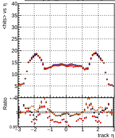
mean hits DQM TT ORIGINAL layerProcv2 DQM TT MODIFIED layerProcv2_windows DQM TT MODIFIED layerProcv2_windows_hits
