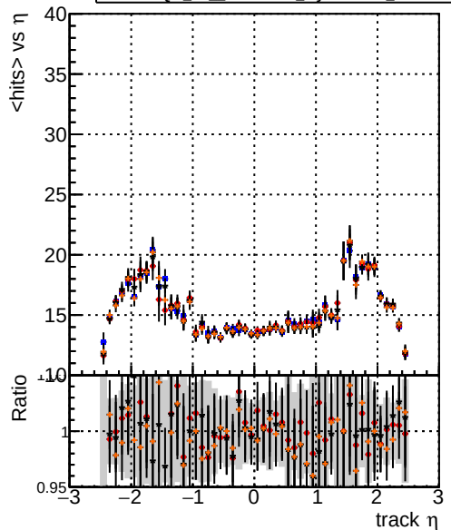
mean hits vs \eta Legend: DQM TT ORIGINAL DQM TT MODIFIED layerProc2 DQM TT MODIFIED layerProc2_windows DQM TT MODIFIED layerProc2_windows_hits
