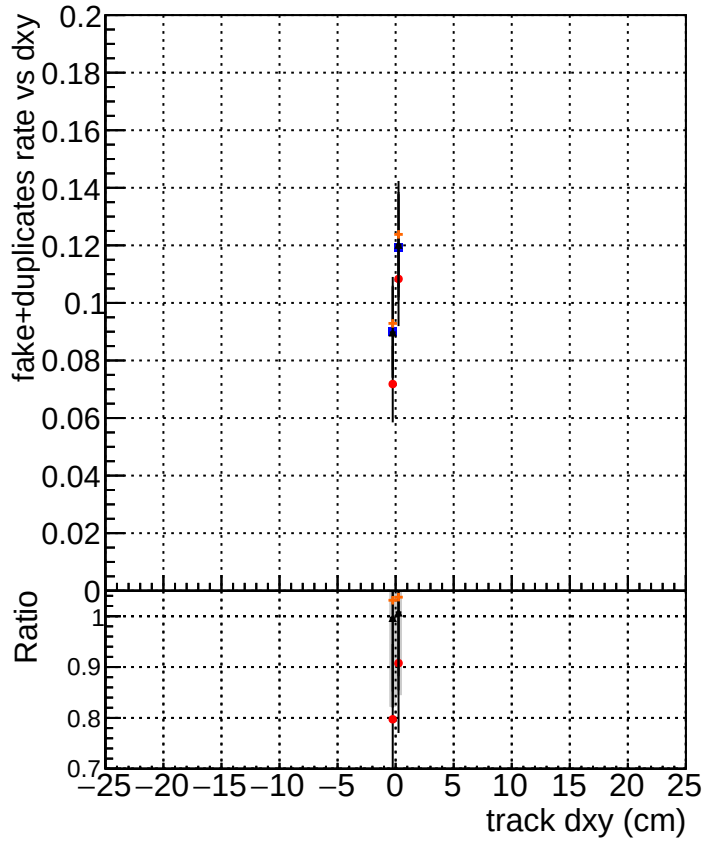
DQM_TT_ORIGINAL DQM_TT_MODIFIED_layerProcv2 DQM_TT_MODIFIED_layerProcv2_windows DQM_TT_MODIFIED_layerProcv2_windows_hits
