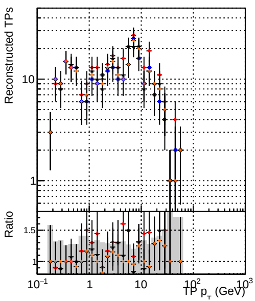
● DQM TT ORIGINAL layerProc2 ● DQM TT MODIFIED layerProc2 ● DQM TT MODIFIED layerProc2_windows ● DQM TT MODIFIED layerProc2_windows_hits
