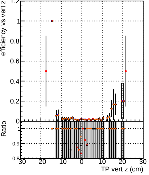
Efficiency vs TP vert z (cm) Legend: DQM TT ORIGINAL DQM TT MODIFIED layerProcv2 DQM TT MODIFIED layerProcv2_windows DQM TT MODIFIED layerProcv2_windows_hits
