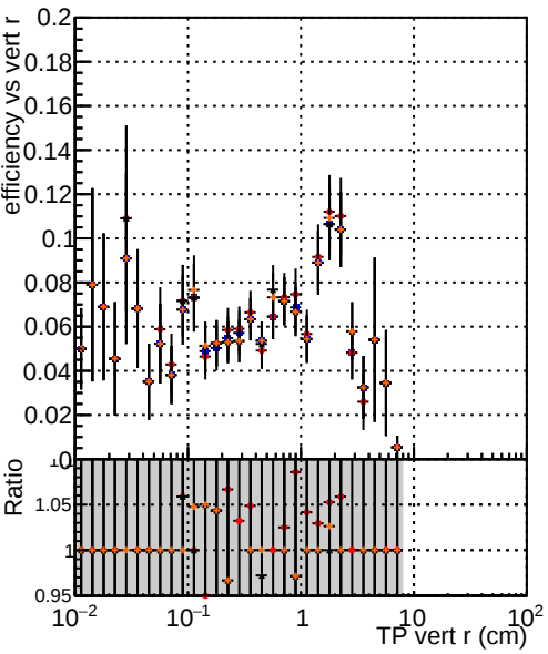
Efficiency vs vertpos —●— DQM TT ORIGINAL —●— DQM TT MODIFIED layerProcv2 —●— DQM TT MODIFIED layerProcv2_windows —●— DQM TT MODIFIED layerProcv2_windows_hits
