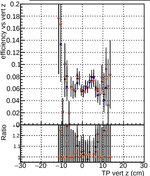
Efficiency vs vertpos —●— DQM TT ORIGINAL —●— DQM TT MODIFIED layerProcv2 —●— DQM TT MODIFIED layerProcv2_windows —●— DQM TT MODIFIED layerProcv2_windows_hits
