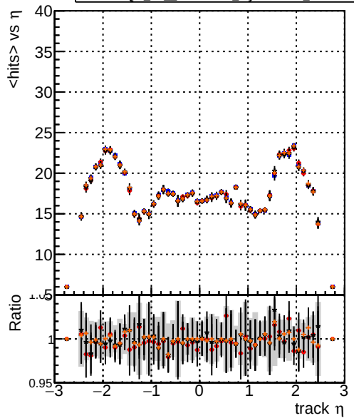
mean hits DQM TT ORIGINAL layerProcv2 DQM TT MODIFIED layerProcv2_windows DQM TT MODIFIED layerProcv2_windows_hits
