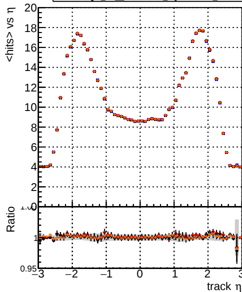
mean hits DQM TT ORIGINAL DQM TT MODIFIED layerProcv2 DQM TT MODIFIED layerProcv2_windows DQM TT MODIFIED layerProcv2_windows_hits
