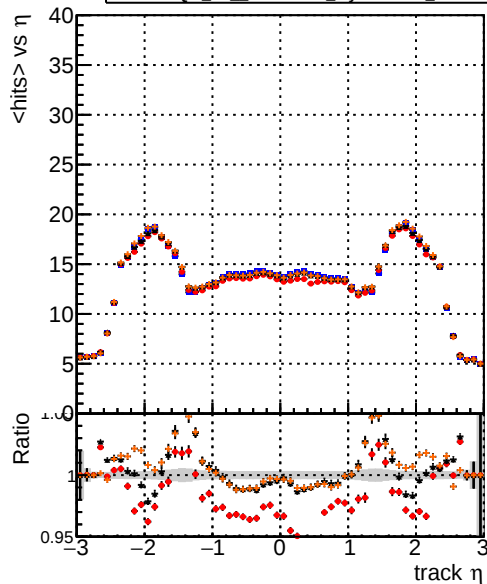
mean hits DQM TT ORIGINAL layerProcv2 DQM TT MODIFIED layerProcv2 DQM TT MODIFIED layerProcv2_windows DQM TT MODIFIED layerProcv2_windows_hits
