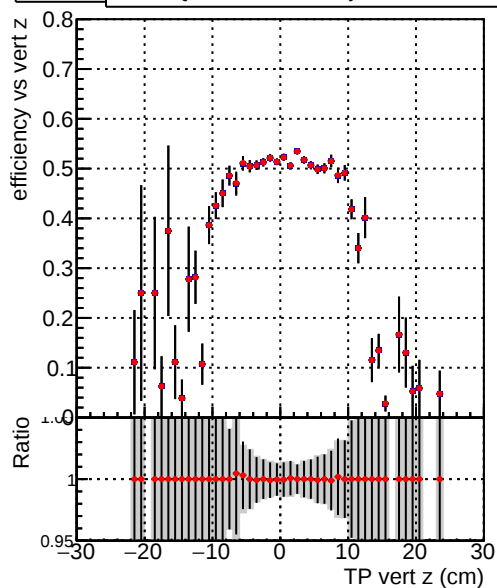
Efficiency vs vert z — DQM_TT_ORIGINAL — DQM_TT_MODIFIED_layerProcV2_PRVersion
