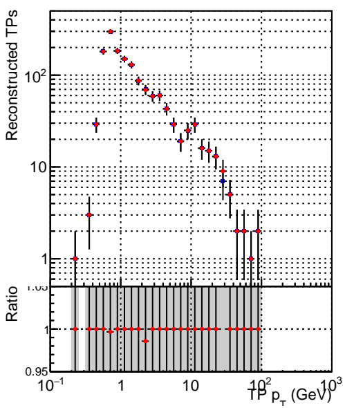
■ DQM_TT_ORIGINAL ◆ DQM_TT_MODIFIED_layerProcV2_PRVersion
