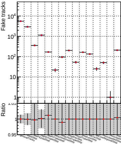
Numbe DQM_TT_MODIFIED_layerProcV2_PRVersion 1 1 2 2 3 3 4 4 5 5 6 6 7 7 8 8 9 9 10 10 11 11 12 12 13 13 14 14 15 15 16 16 17 17 18 18 19 19 20 20 21 21 22 22 23 23 24 24 25 25 26 26 27 27 28 28 29 29 30 30 31 31 32 32 33 33 34 34 35 35 36 36 37 37 38 38 39 39 40 40 41 41 42 42 43 43 44 44 45 45 46 46 47 47 48 48 49 49 50 50 51 51 52 52 53 53 54 54 55 55 56 56 57 57 58 58 59 59 60 60 61 61 62 62 63 63 64 64 65 65 66 66 67 67 68 68 69 69 70 70 71 71 72 72 73 73 74 74 75 75 76 76 77 77 78 78 79 79 80 80 81 81 82 82 83 83 84 84 85 85 86 86 87 87 88 88 89 89 90 90 91 91 92 92 93 93 94 94 95 95 96 96 97 97 98 98 99 99 100 100
