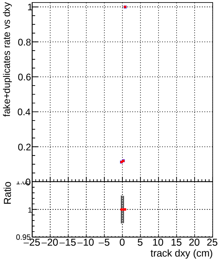
DQM_TT__ORIGINAL DQM_TT__MODIFIED_layerProcv2_PRVersion
