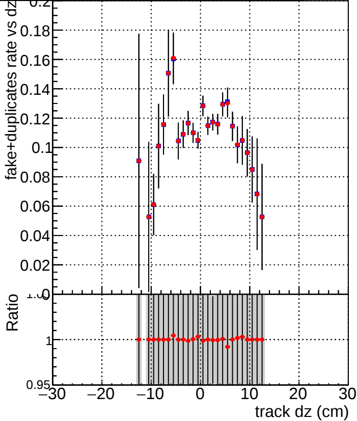
DQM_TT__ORIGINAL DQM_TT__MODIFIED_layerProcv2_PRVersion
