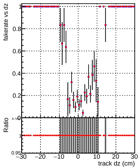
Fake rate vs dz —•— DQM TT ORIGINAL —•— DQM TT MODIFIED_layerProcV2_PRVersion
