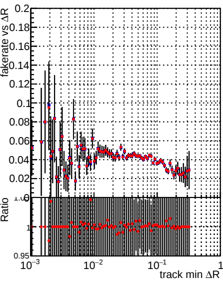
DQM_TT_ORIGINAL DQM_TT_MODIFIED_layerProcv2_PRVersion
