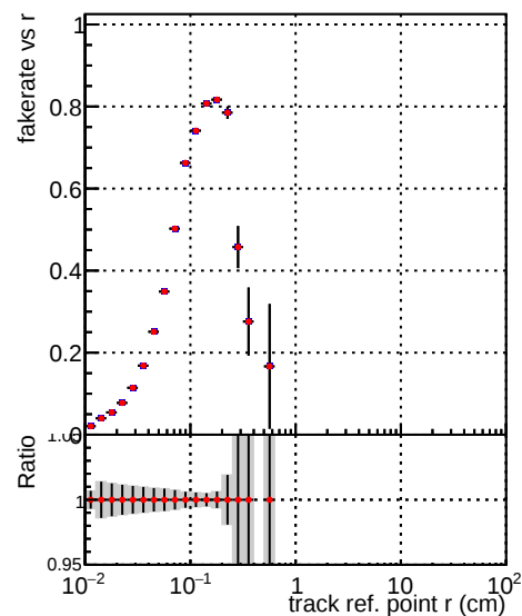
—●— DQM_TT_ORIGINAL —●— DQM_TT_MODIFIED_layerProcV2
