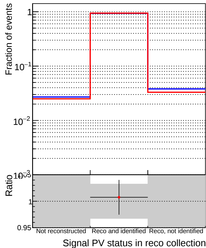
■ DQM_TT_ORIGINAL ● DQM_TT_MODIFIED_layerProcv2
