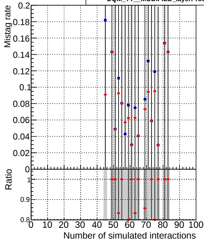
■ DQM_TT_ORIGINAL ● DQM_TT_MODIFIED_layerProcv2
