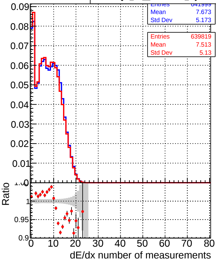
■ DQM_TT_ORIGINAL ● DQM_TT_MODIFIED_layerProcv2
