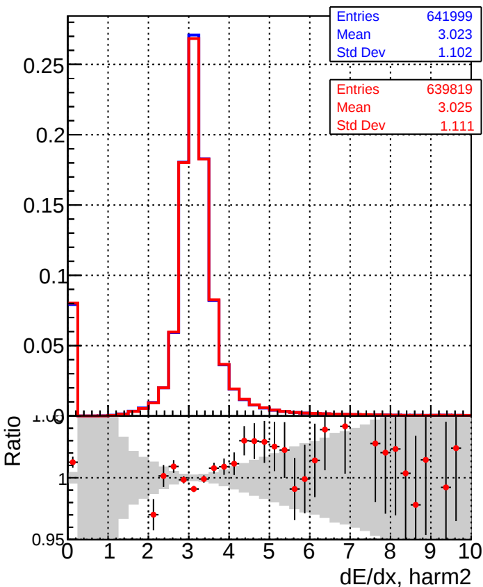
■ DQM_TT_ORIGINAL ● DQM_TT_MODIFIED_layerProcv2
