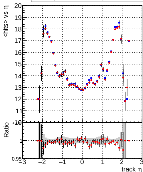
— DQM_TT_ORIGINAL — DQM_TT_MODIFIED_layerProcV2
