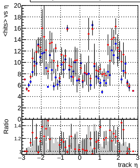
mean hits — DQM_TT_ORIGINAL — DQM_TT_MODIFIED_layerProcV2
