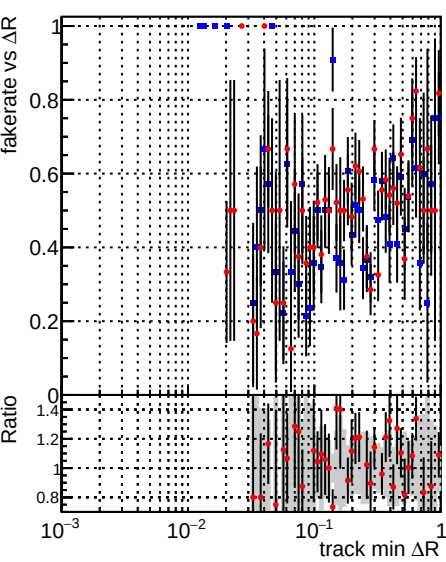
DQM_TT_ORIGINAL DQM_TT_MODIFIED_layerProcv2
