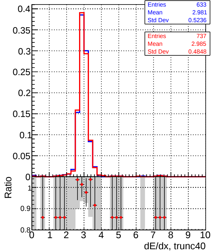
dE/dx estimator 2
