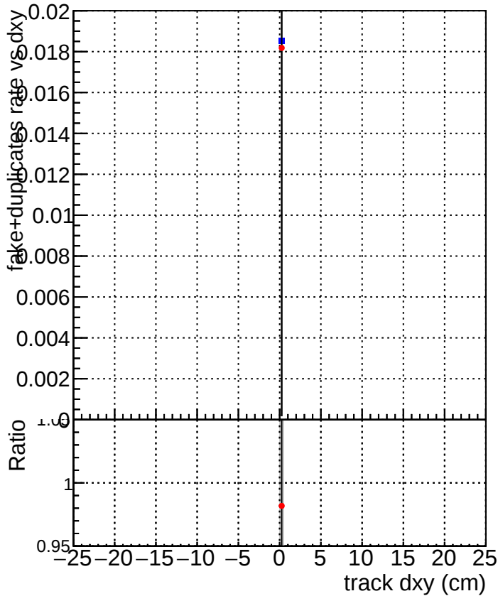
DQM_TT_ORIGINAL DQM_TT_MODIFIED_layerProc2
