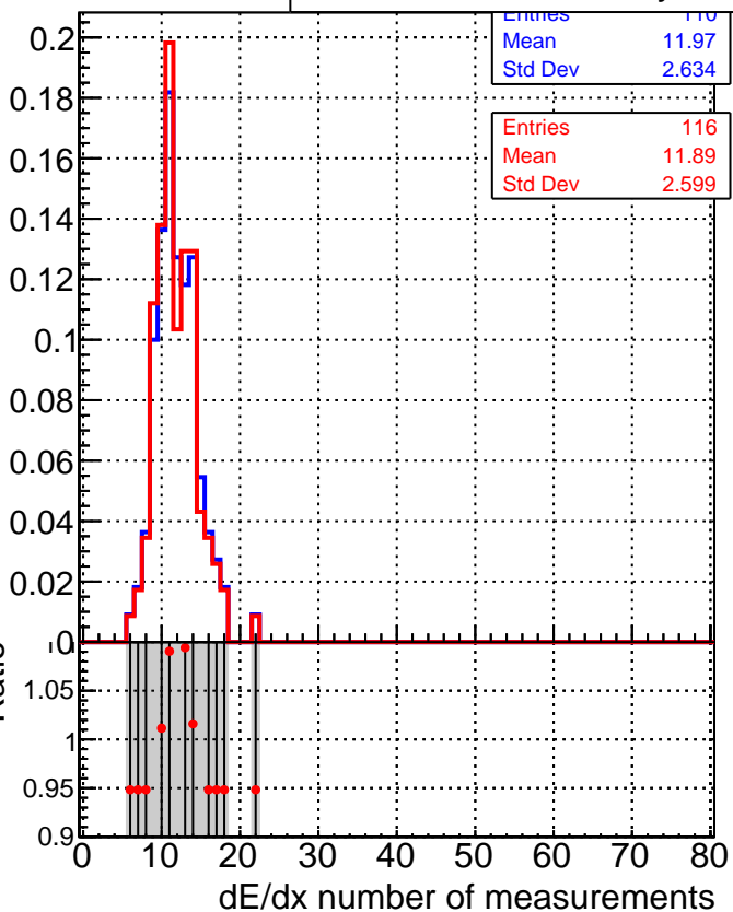
■ DQM_TT_ORIGINAL ● DQM_TT_MODIFIED_layerProc2
