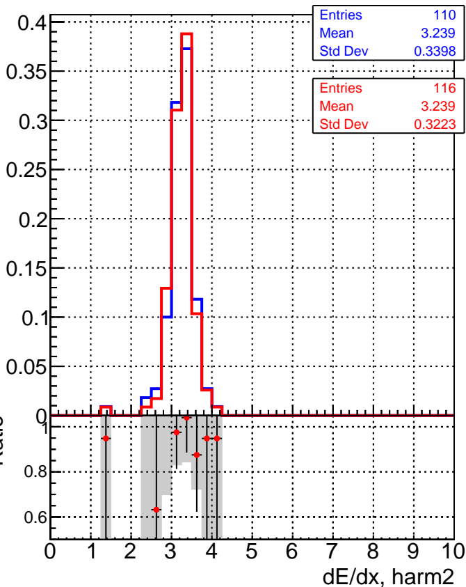
■ DQM_TT_ORIGINAL ● DQM_TT_MODIFIED_layerProc2
