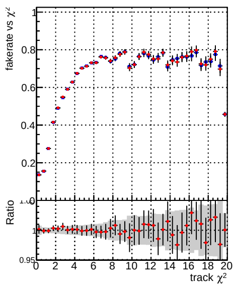
Fake rate vs. —●— DQM TT ORIGINAL —●— DQM TT MODIFIED layerProcV2
