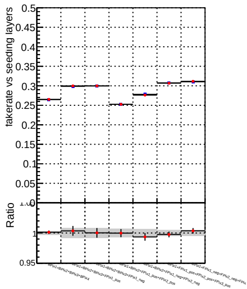
Fake rate vs. —●— DQM TT ORIGINAL —●— DQM TT MODIFIED layerProcV2
